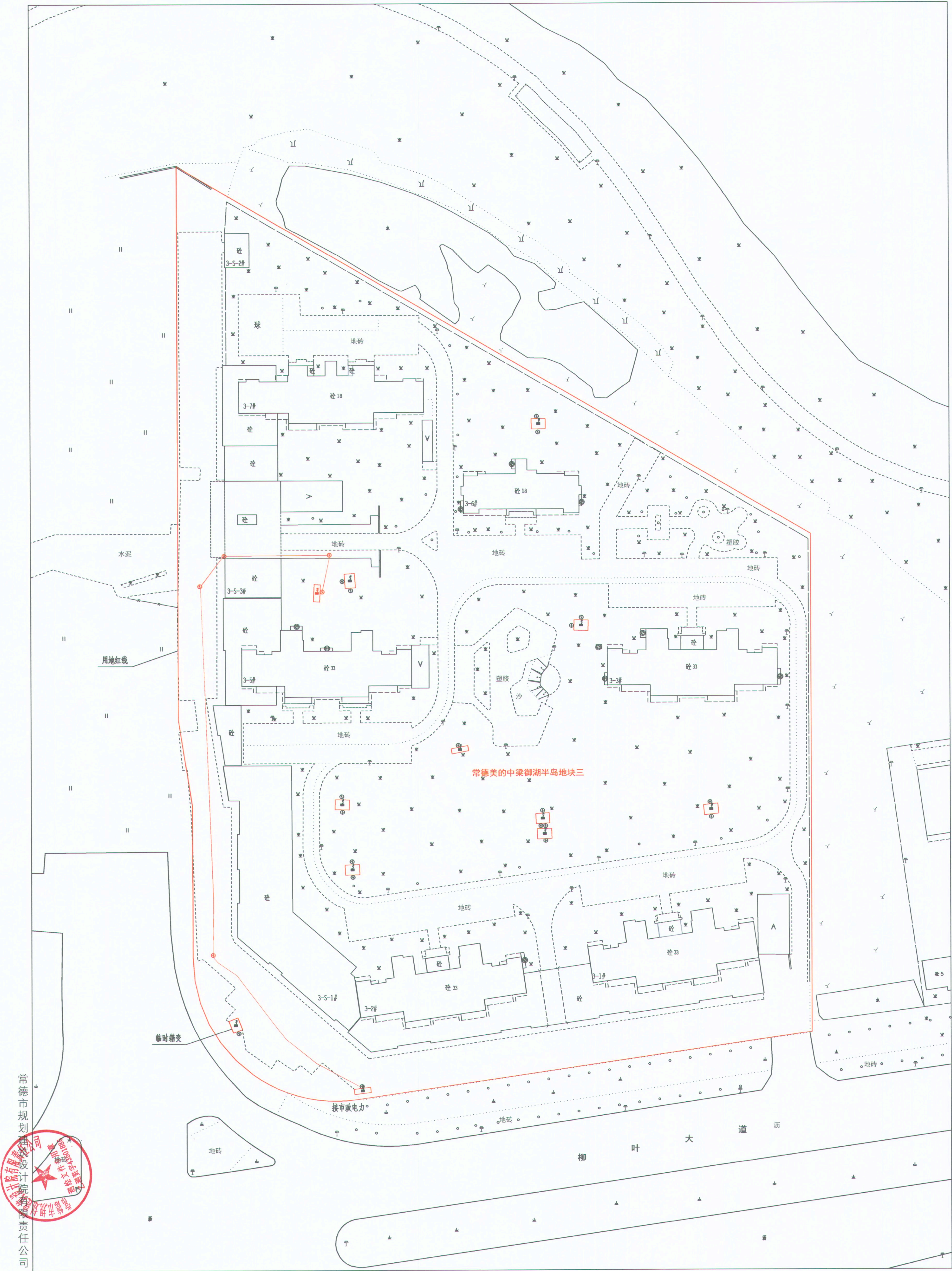
常德美的中梁御湖半岛地块三供配电设备及电力管线平面公示图
